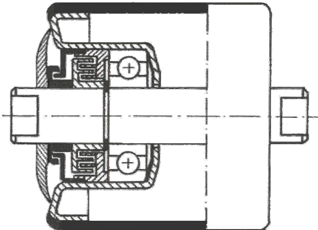
Offshore toepassing met lipafdichting
