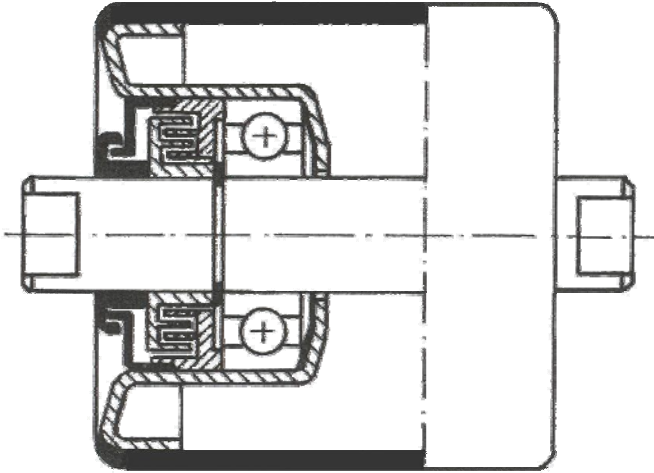
Type RSND met primer coating Type RSNE met epoxy coating
